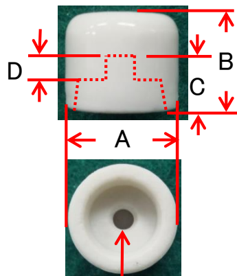
ネジ孔 M3
